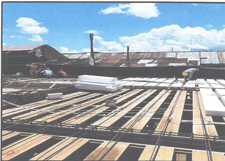
ENCOFRADO Y COLOCACION DE ACERO EN LOSA ALIGERADA EN CONTINGENCIA - ISLANDIA.
