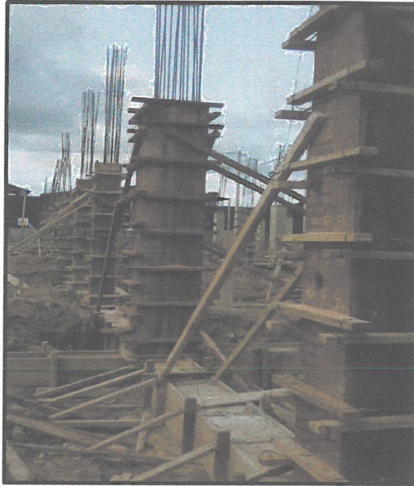
ENCOFRADO DE COLUMNAS EN C.S ISLANDIA.
